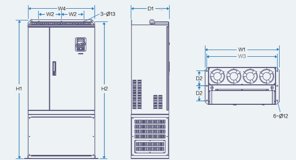
Напольный монтаж преобразователей 350—500кВт
