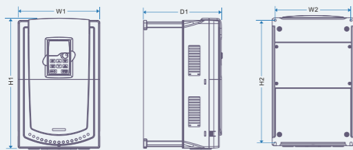
Схема установки для ПЧ 18—55кВт
