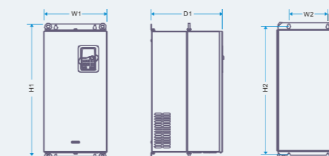
Фланцевый монтаж преобразователей 132 ~ 200кВт
