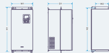
Фланцевый монтаж преобразователей 18 ~ 55кВт
