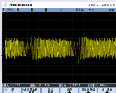
Форма тока в режиме векторного управления без обратной связи с полной нагрузкой на частоте 50 Гц.
